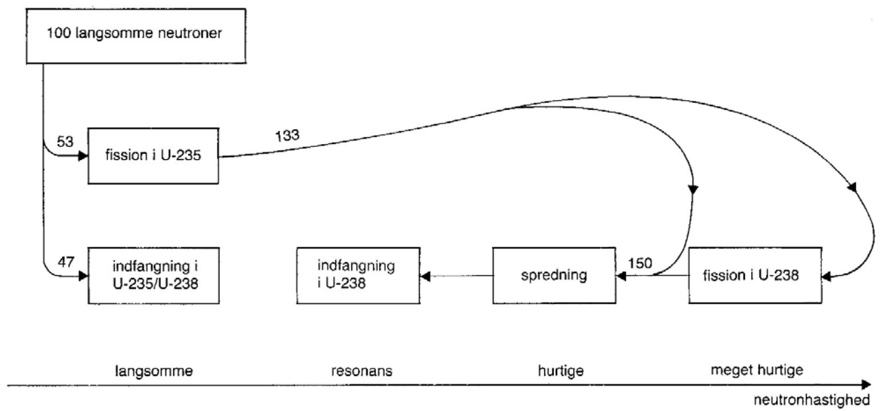
Figur 5.4 100 neutroners skæbne i naturligt uran.
