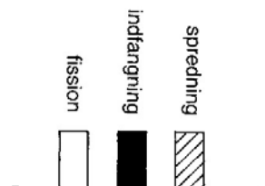
Figur 5.3 Reaktionstværsnit for en neutrons møde med en urankerne.
