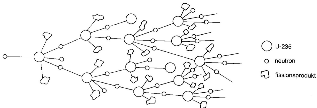
Figur 5.1 Kædereaktion ved fission
