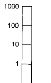
Figur 5.3 Reaktionstværsnit for en neutrons møde med en urankerne.
