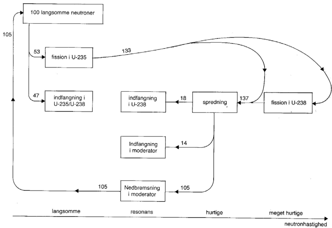
Figur 5.6 100 neutroners skæbne i naturligt uran med moderator.
