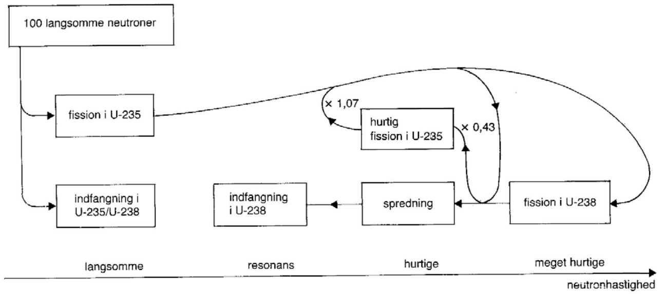
Figur 5.7 100 neutroners skæbne i uran beriget til 25% U-235.
