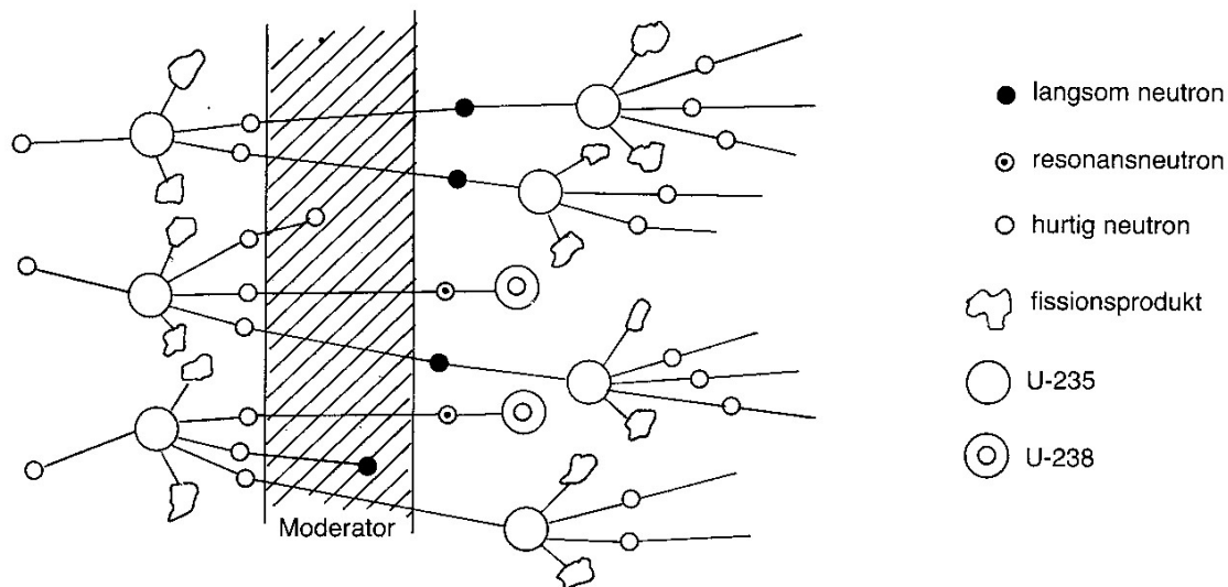
Figur 5.5 Kædereaktion i naturligt uran med moderator.
